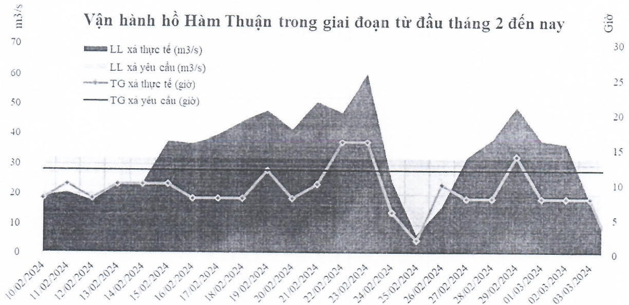
Hình 1. So sánh thực tế vận hành xả phát điện hồ Hàm Thuận với quy định của QTVH
